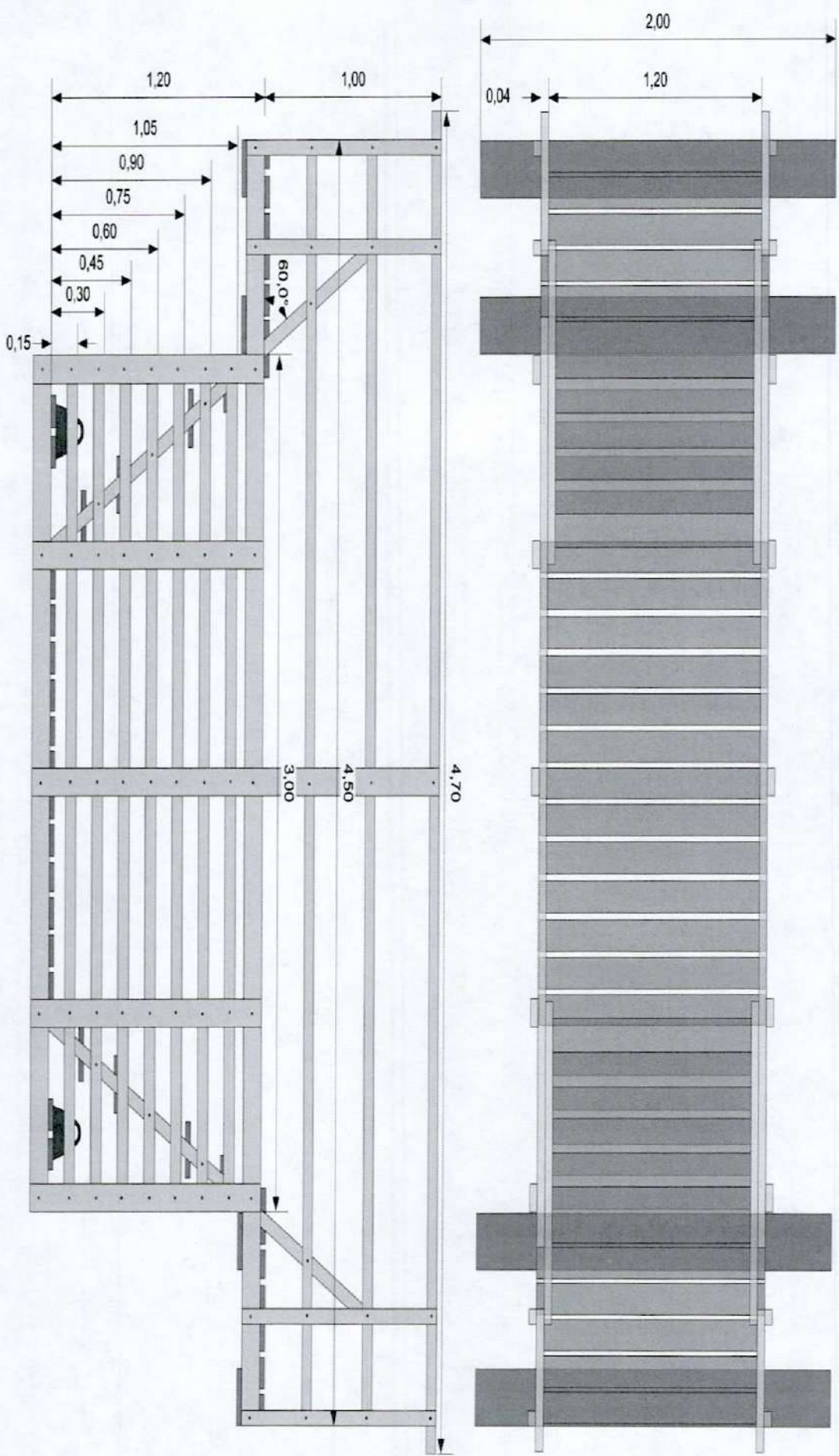
Чертеж конструктивной мостков для Крещенских купаний на водных объектах (вариант 2)
